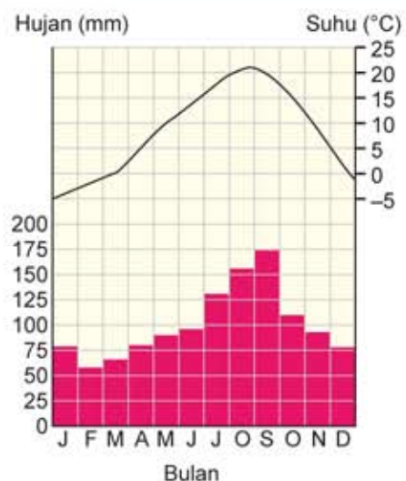
Graf 7.4 Suhu dan hujan bulanan di Hakodate, Jepun (Sumber: Climate-Data.org, 2016)
